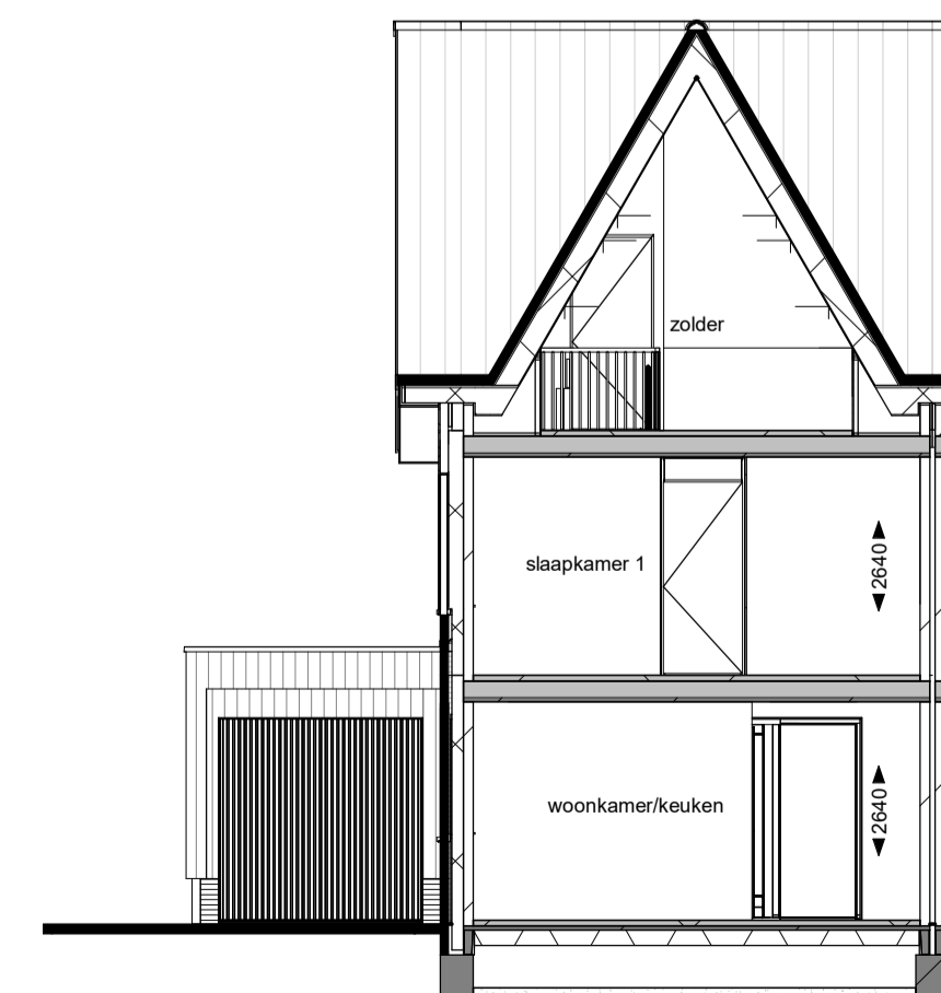
Doorsnede B
