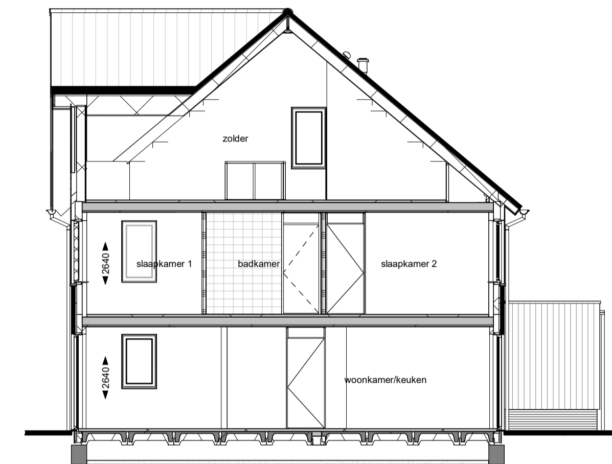
Doorsnede A
