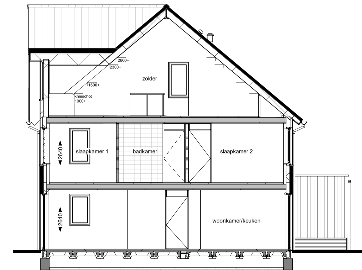
Doorsnede A
