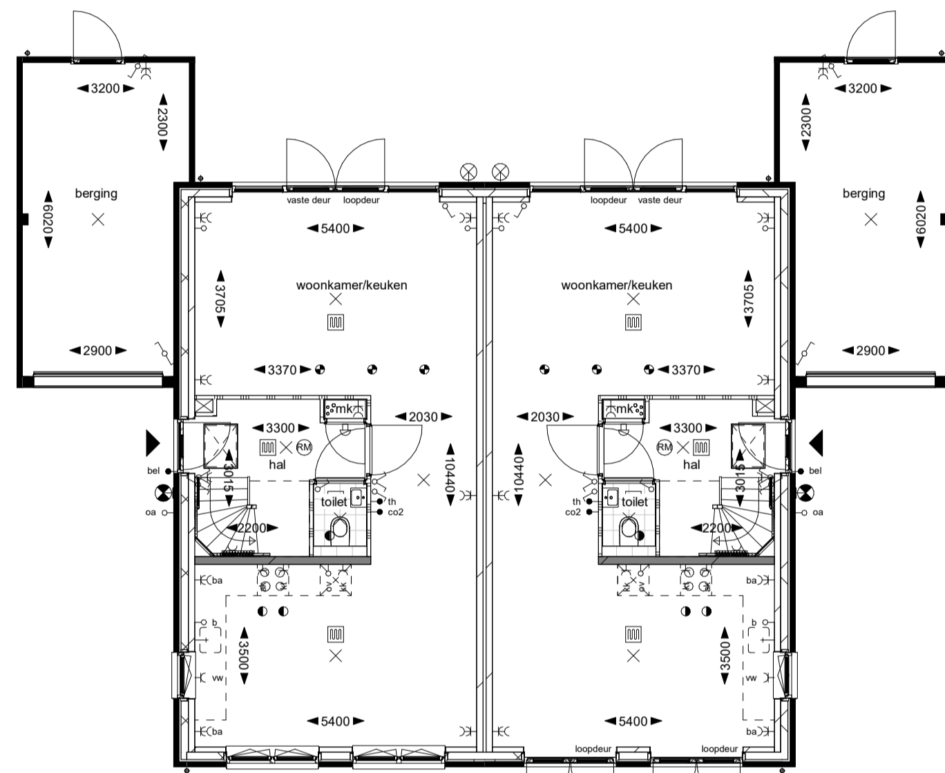
Begane grond
