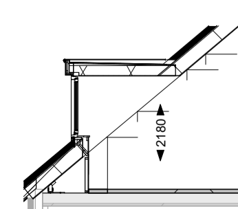
Doorsnede
