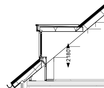
Doorsnede
